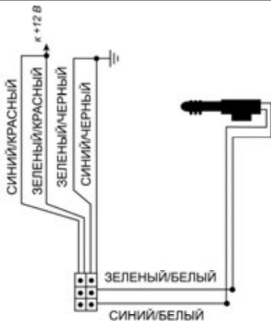
Схема 6. Установка дополнительных электроприборов
